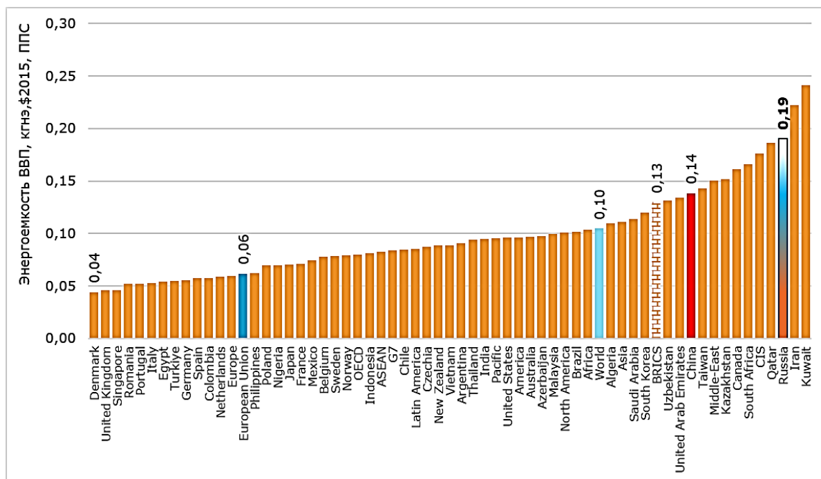
Рисунок 3.6 Россия в мировом рейтинге по энергоемкости в 2025 г.
